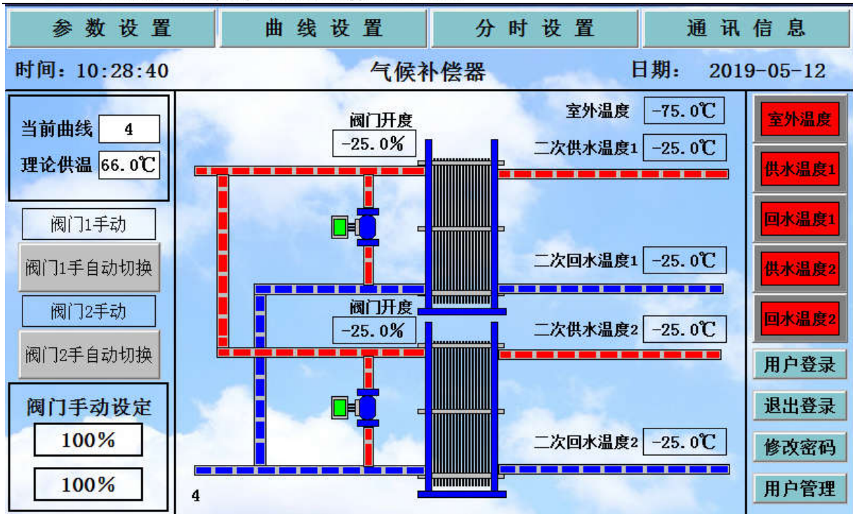
图 9. 阀门旁通安装主画面
